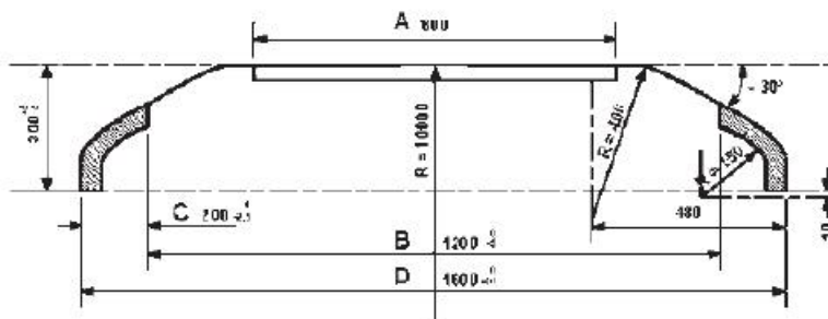
Профил главе пантографа
